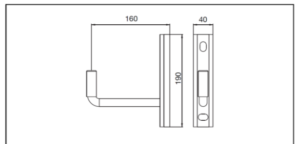
Mocowanie ścienne
