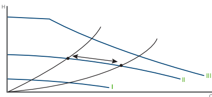
Rys. 10 Trzy nastawy charakterystyki stałej/prędkości stałej
