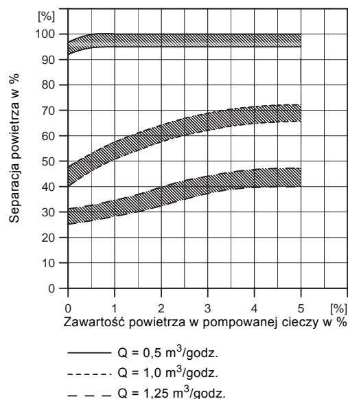
Rys. 20 Separacja powietrza
