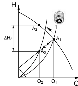
Rys. 12 Praca pompy przy regulacji ciśnienia proporcjonalnego
