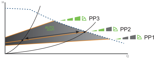
Rys. 8 Trzy charakterystyki/nastawy proporcjonalnej regulacji ciśnienia
