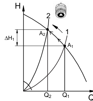
Rys. 11 Pompa nieregulowana
