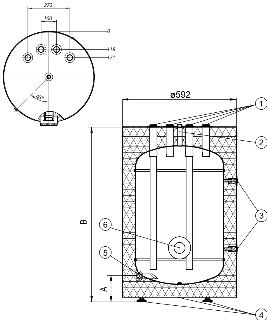
Устройство буферного накопителя SVK 100
