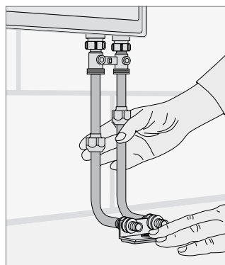
Rys. 14-7 Zakładanie kątowych garniturów przyłączyowych
