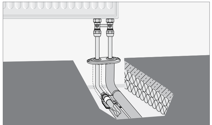
Rys. 16-6 Podwójna rozeta na podłodze
