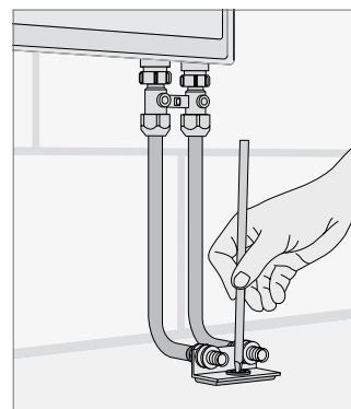
Rys. 14-8 Zaznaczanie otworów do nawiercenia pod jednostkę mocującą
