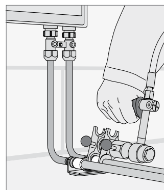
Rys. 14-10 Wykonanie połączenia typu tuleja zaciskowa
