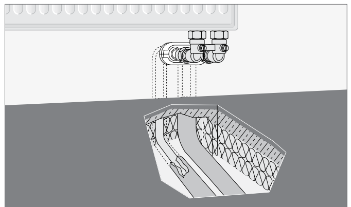
Rys. 16-7 Podwójna rozeta na ścianie
