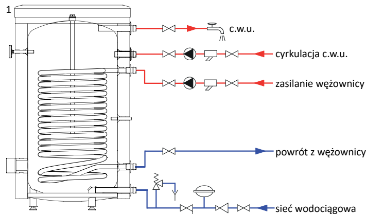
Rys. 9 Schemat instalacyjny zasobnika W-E 100.81, W-E 150.81 z jedną węzownicą MEGA.
