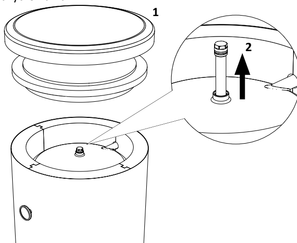
Rys. 10 Wymiana ochronnej anody magnezowej.
