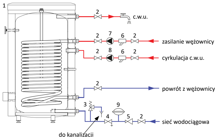
Rys. 8 Schemat instalacyjny zasobnika W-E 125.81 z jedną węzownicą MEGA.
