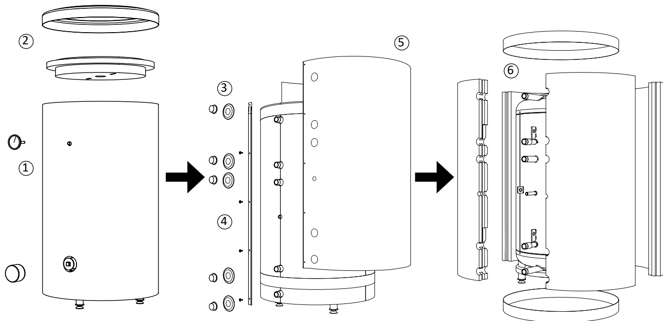
Rys. 7 Demontaż obudowy i izolacji termicznej.
