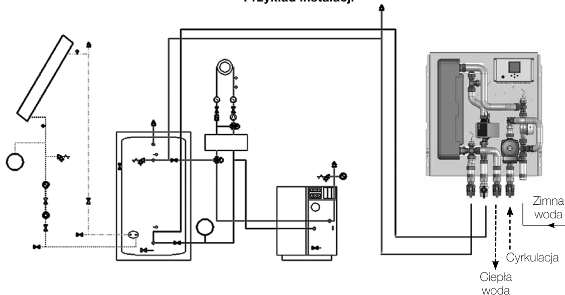
Przykład instalacji
