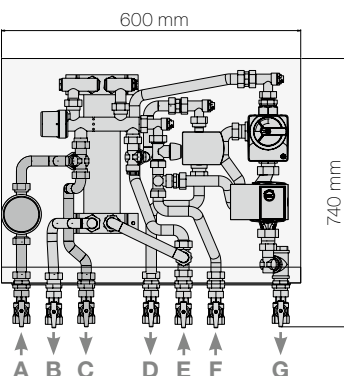
Wymiary standardowego wyposażenia Logotermy Wenus.
