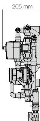
Wymiary standardowego wyposażenia Logotermy Wenus.
