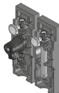
Grupa pompowa bez mieszacza V-UK
