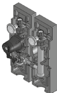
Grupa pompowa z mieszaczem V-MK
